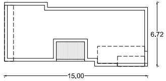
[PLANTA DE COBERTURA]
