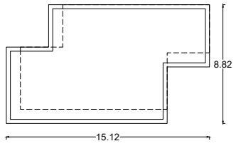
[PLANTA DE COBERTURA]
